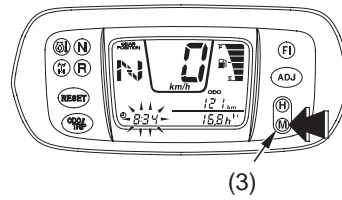
(3) minuuttien valintapainike
