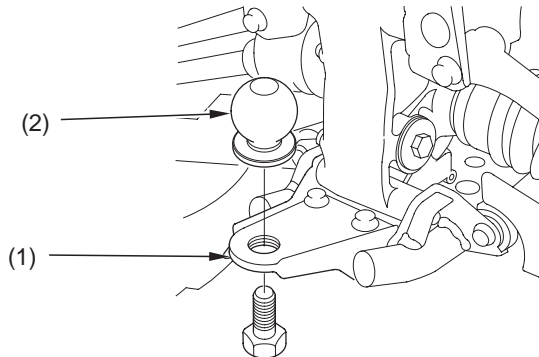
(1) vetonupin kiinnike
