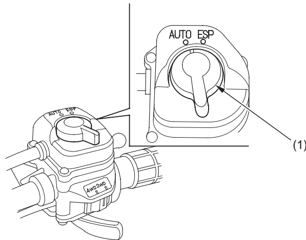
(1) vaihteiston valintakytkin
