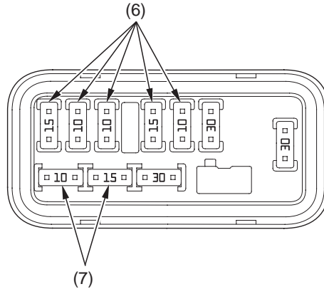
(6) käyttösulake
